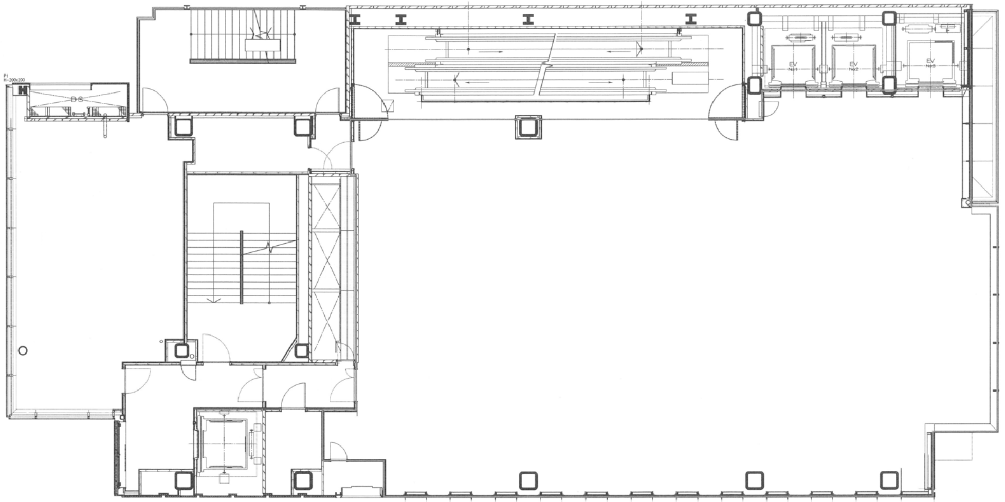
2階平面図
